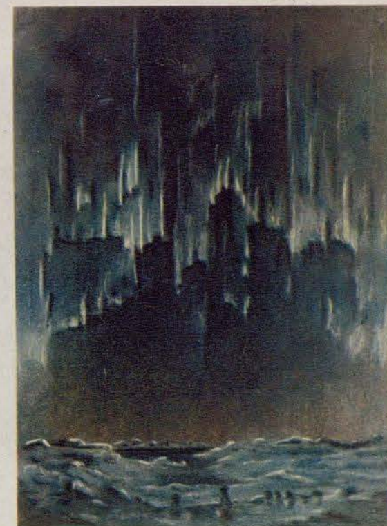
Полярное сияние «Драпри».
