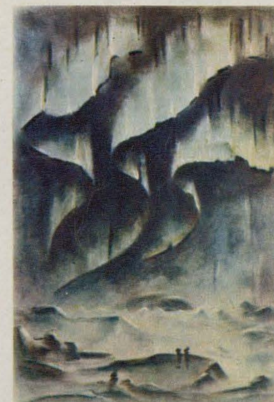
Полярное сияние «Занавес».
