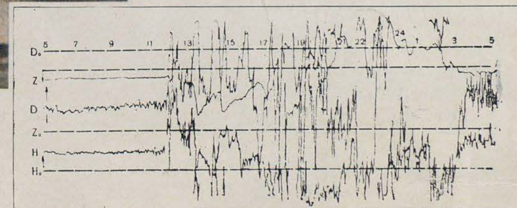
Запись поля магнитной бури, во время которой яркое полярное сияние наблюдалось и в южных широтах.
