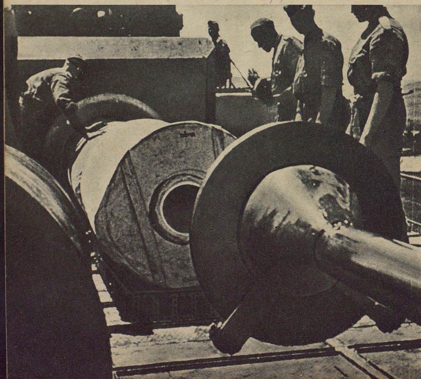
Poussoir de chargement et gargousse à l'ouverture de la culasse.
