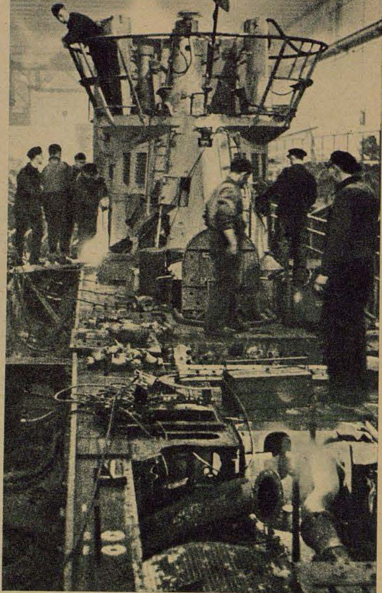
18 Подводницата е на сигурно място въ бронирания докъ. Тукъ се отстраняватъ всички повреди до най-малката, и дружини докови работници извършватъ поправки и подобрения, наложени се отъ природните стихии или неприятелски действия
