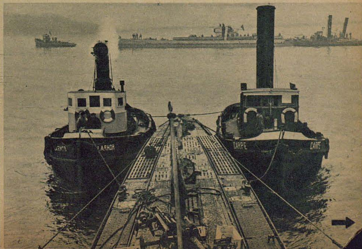
13 Отъ всички люкове се изважда инвентара на подводницата. Машинни части, останали припаси, бельо, сандъци и сандъчета! Смутие изкарва всички сѣдини отъ кухнята сжщо навънъ
