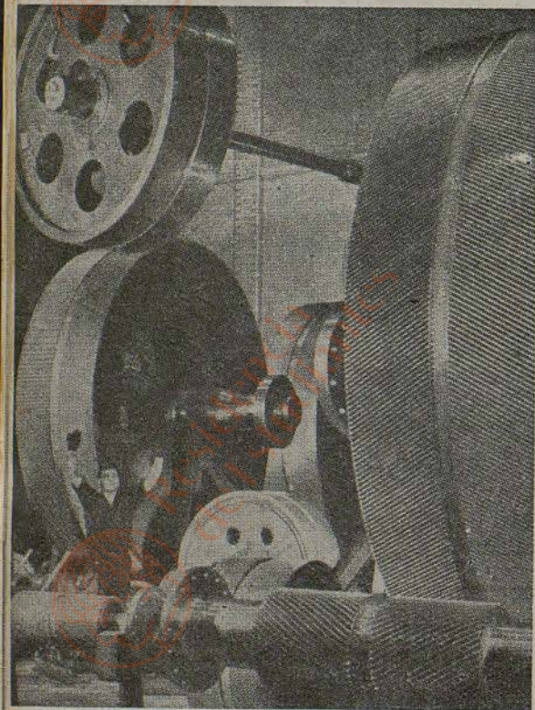
Engranajes contruidos en Estados Unidos para los buques de guerra.—(Foto CIFRA.)
