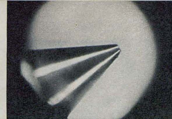
Под микроскопом — одна из корундовых игл, изготовленных в Нииалмаз по заказу группы реставрации.
