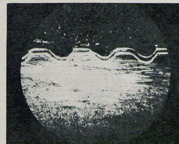
Поперечный срез пластинки под микроскопом. Эти канавки запечатлели голос Ленина.
