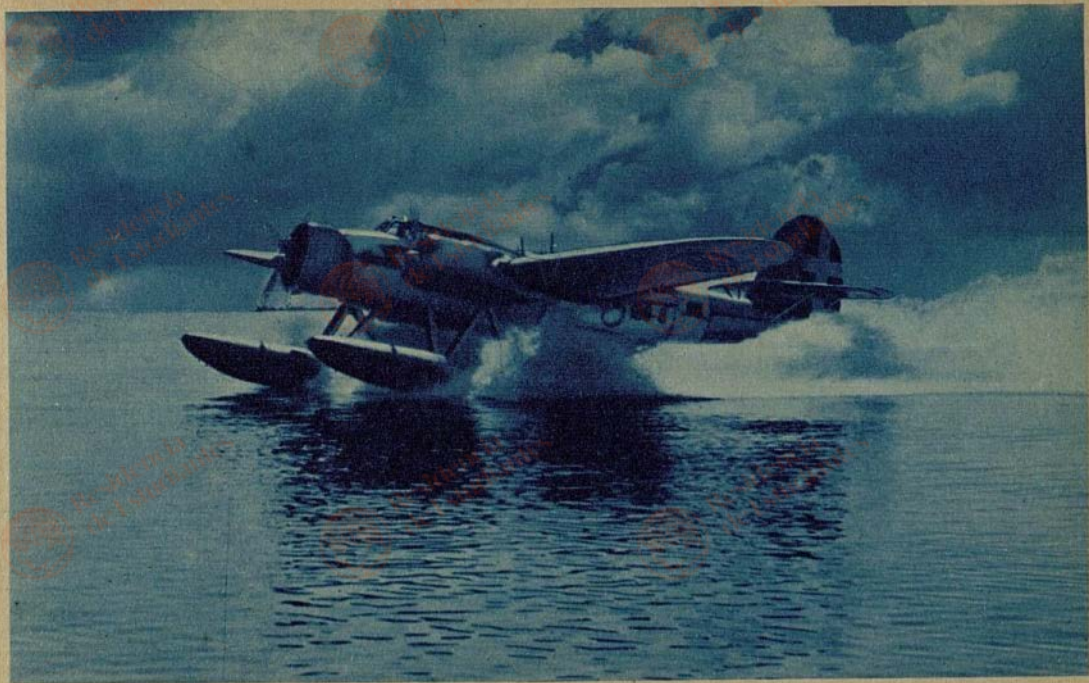
Il decollo di un nostro "Atrone,, da ricognizione marittima
