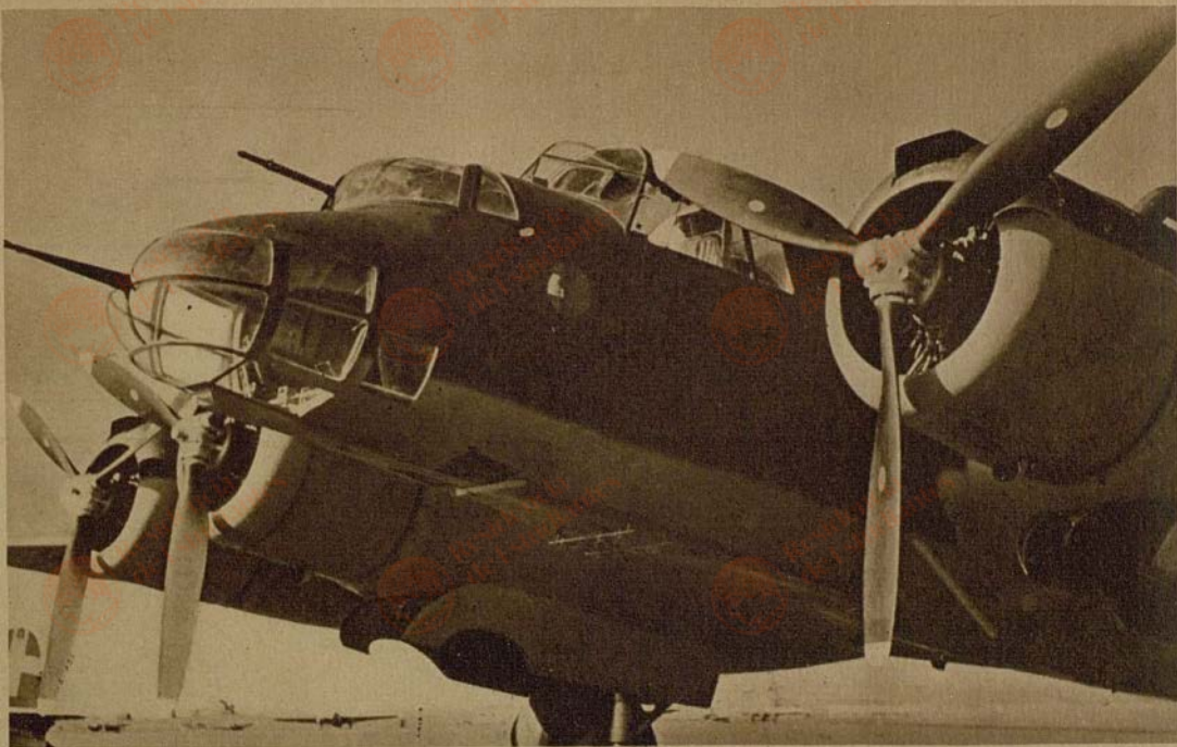
Il "P. 108", visto di fronte
