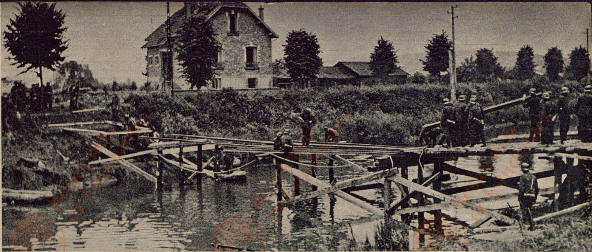
14 h. 15: Toutes les palées sont en place. Les premiers madriers sont amenés...
