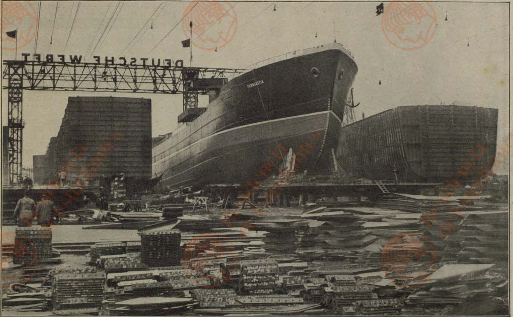
Rechts: So war es früher: Schiffsleib an Schiffsleib, untätig Monate, Jahre; ein Kriechhof der ganze Hafen
