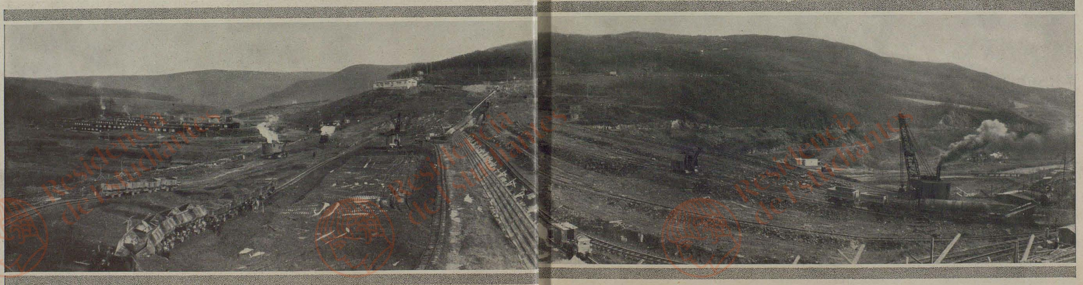
Das untere Panorama zeigt (links) das aus 14 Untertunftshäusern bestehende Waldlager Schwammenauel für die an der Baustelle wohnenden Gefolgschaftsmitglieder. Auf der Bergeshöhe (halblinks) liegt das örtliche Baubüro. Im Vordergrund (Mitte) ist der Sperrdamm mit den einzelnen Stützkörpern, vom linken Hang aus gesehen.
