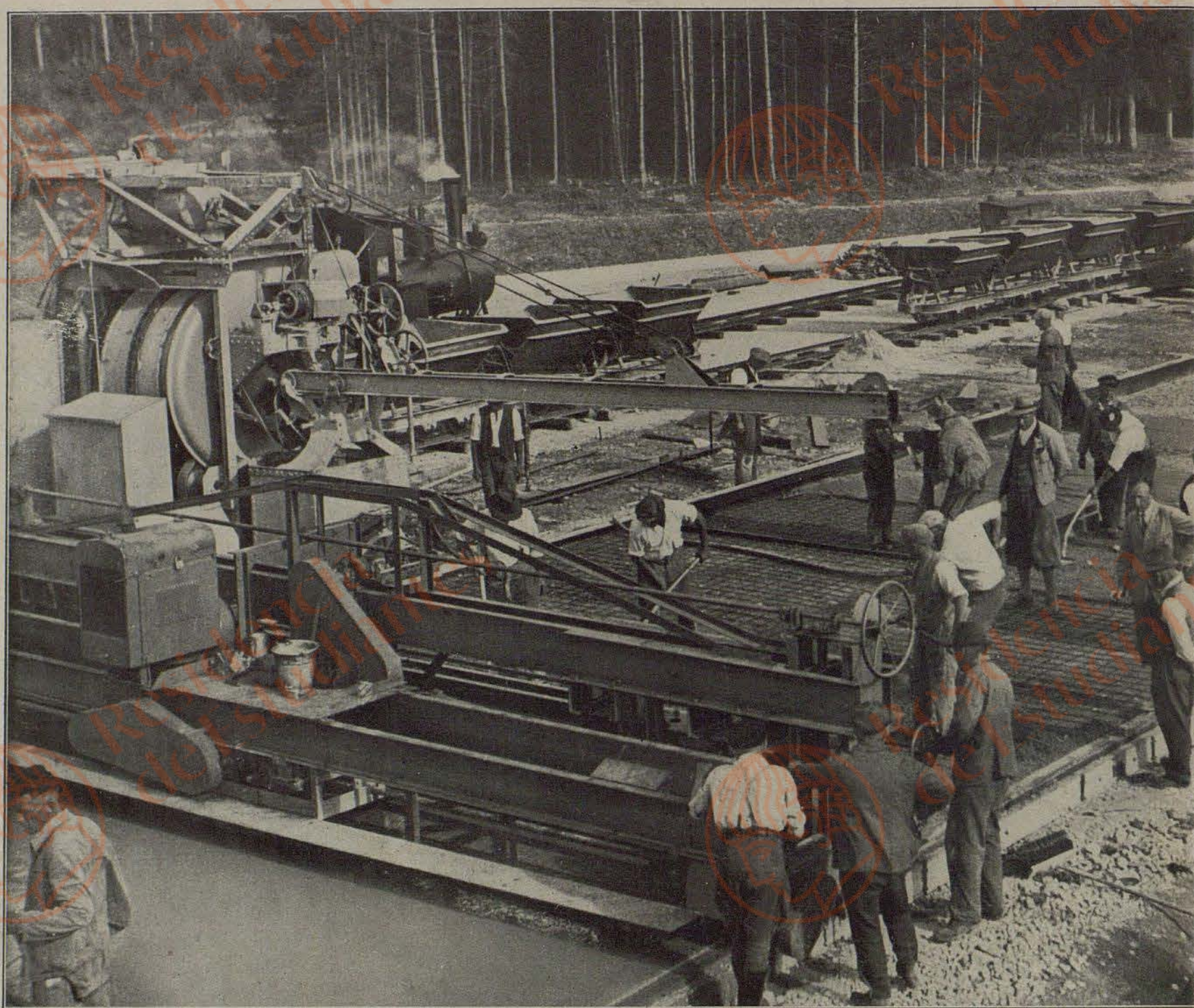
So entstehen die Reichsautobahnen Nach der schnurgeraden Ebnung erhält die Straße ihre Vede Ganz neuartige Maschinengiganten des modernen Straßenbaues ergänzen die schaffende Kraft
