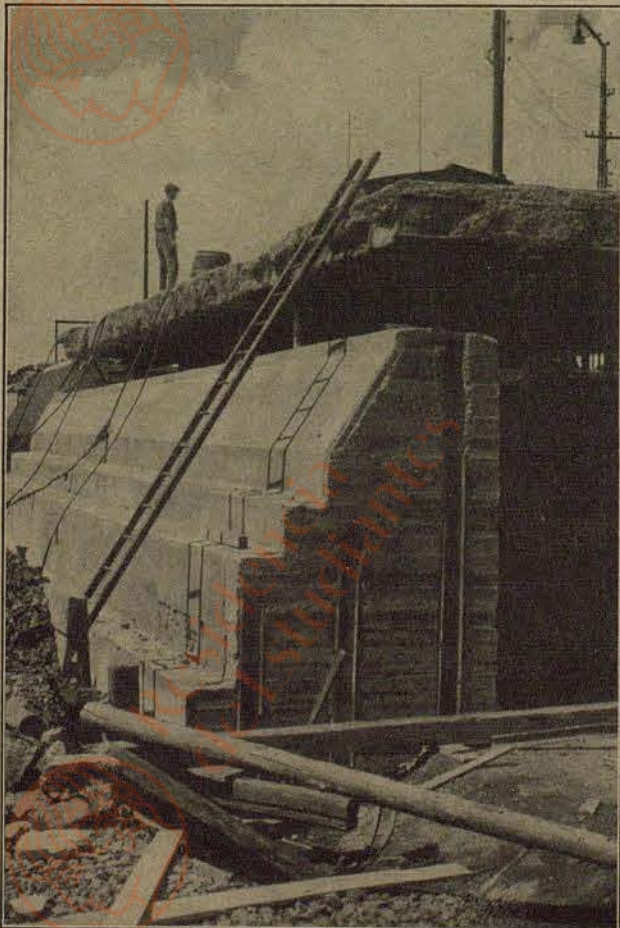
Hebungen im saarländischen Grubenjunktionsgebiet. Eine 130 m lange Brücke wird um 4 m gehoben.
