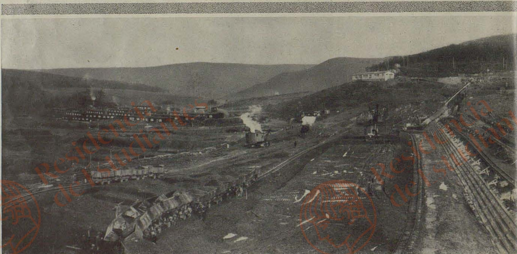
Gesamtbild der Baustelle mit dem Sperrdamme, vom linken Hang aus gesehen. Auf der Bergeshöhe (halbwegs) liegt das örtliche Baubüro. Im Vordergrund gleiten, in dessen Mitte die Spundwand zu sehen ist.
